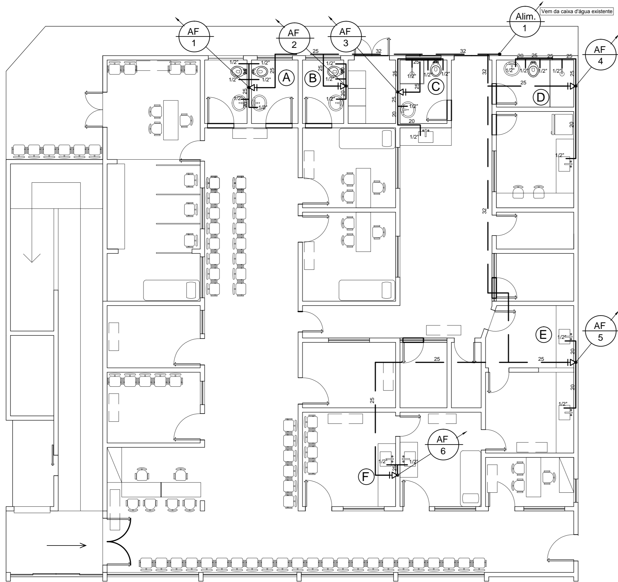
PLANTA BAIXA - TÉRREO HIDRÁULICA 1:75
